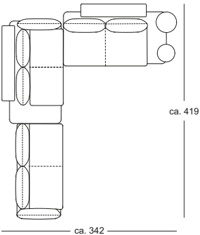
A-ASO 515/185 li. RA-A-ASO 515/185 A-SOB-ABL 515/203 re. UE-RA-A-SOB-ABL 515/203 re. Schap asymmetrisch Koppelrug re. ARB-ABL 515/203 re. UE-RA-ARB-ABL 515/203 re. Schap symmetrisch Tableau hoot Tableau metaal
